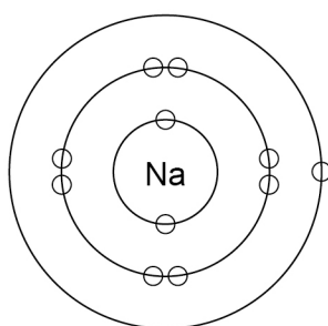
Sodium atom
